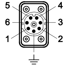
Abbildung 1: Anschlussstecker
