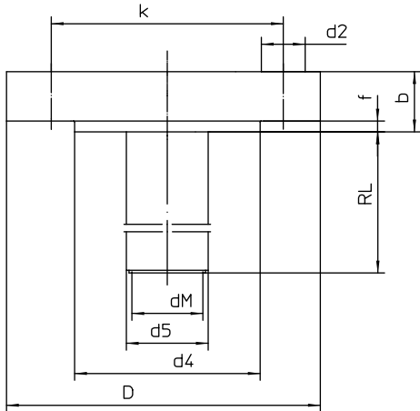
Abmessungen (mm) EN 1092-1
